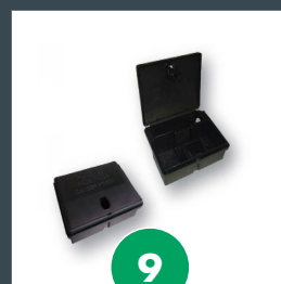
CAIXA PORTA-ISCA (modelo PETI) 40 x 100 x 125 mm
